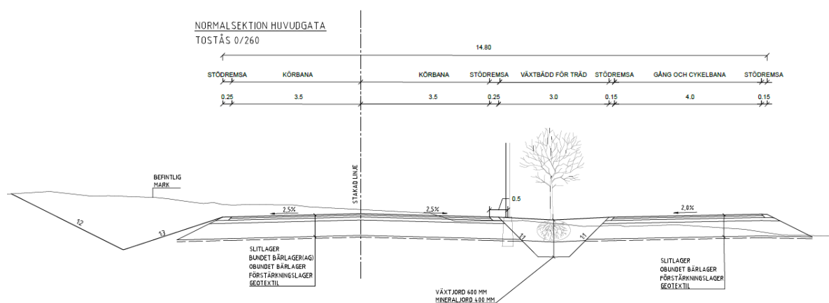
Figur 14. Sektion över huvudgatans utformning.
